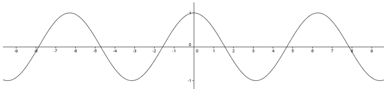
FIGURE – Courbe représentative de la fonction cosinus
